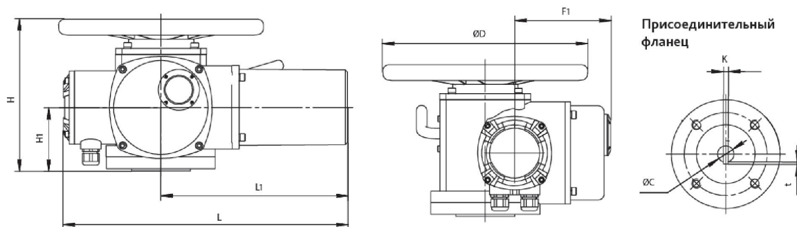
Рис. 1. Габаритные характеристики электроприводов
