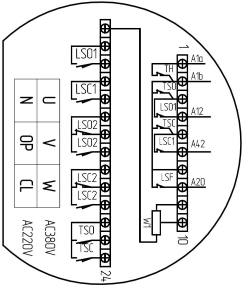
Плата подключения внешних цепей, Вариант 1
