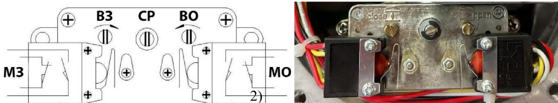
Рис. 5. Блок конечных выключателей
